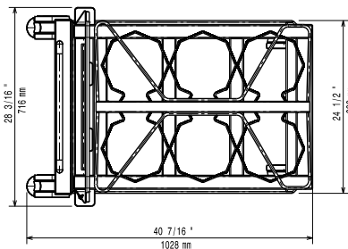
Boven aanzicht
